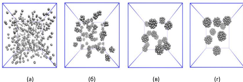
Рис. 1. Визуализация моделей магнитных наночастиц: (а) подвижные одиночные частицы (FF), агрегаты со случайной внутренней конфигурацией частиц, состоящие из (б) 8 (RCC8), (в) 32 (RCC32) и (г) 64 (RCC64) частиц
