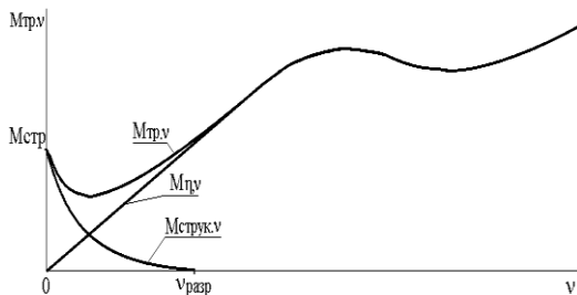
Рис. 1. Изменение M_{\text{тр}}
