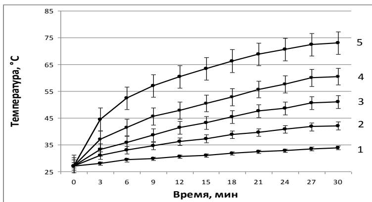
Рис. 6. Зависимость температуры в рабочем зазоре, образованном сменной втулкой (сталь 3, Ra=1,220 мкм) и сменным полюсом (сталь 3; Ra=3,301 мкм) и заполненным магнитной жидкостью типа МКУ 100-40 от времени работы установки, с разными частотами вращения втулки: 1 – 556 об/мин; 2 – 1146 об/мин; 3 – 1793 об/мин; 4 – 2331 об/мин; 5 – 2897 об/мин
