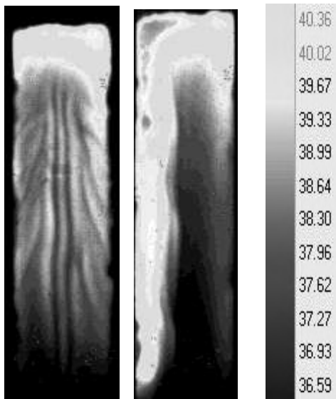
Рис. 2. Термомагнитная конвекция при \Delta T = 18.9 К, H = 34 кА/м и \alpha = 0^0 (слева) и 20^0 (справа)
