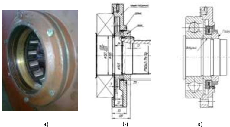
Рис. 3. Крышка подшипника электродвигателя ВАО-630
