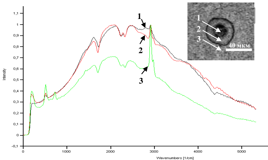
Рис. 4 – Эрозивная структура в виде кольца на катоде и спектры комбинационного рассеяния в разных участках (15 мин, 5 кВ)
