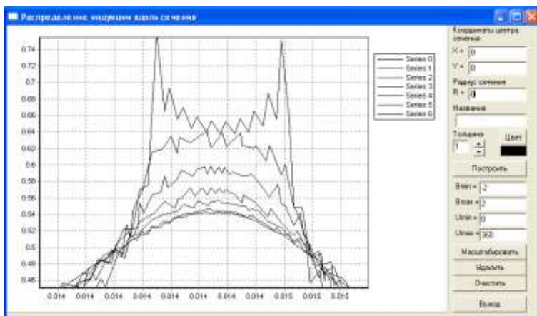
Рис. 6. Кривые распределения индукции в зазоре в нескольких сечениях по высоте зазора под зубом МЖГ
