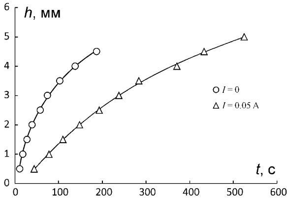
Рис. 2. Экспериментальная зависимость высоты поднятия магнитной жидкости в трубке с песком от времени.
