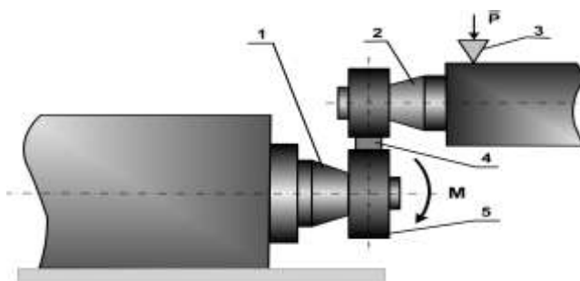
Рис. 2. Упрощенная схема узла трения машины СМТ – 1: 1 – нижний (вращающийся) вал; 2 – верхний (неподвижный) вал; 3 – нагружающее устройство; 4 – образец; 5 – контртело.
