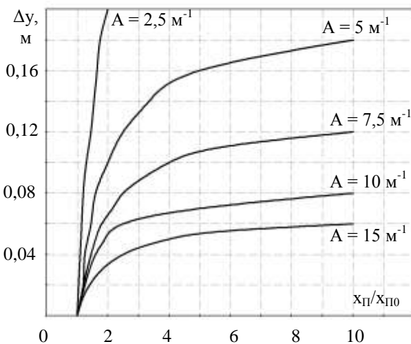
Рис. 2. Профили полюсных наконечников при различных значениях A .
