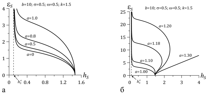
Рис. 2. Фазовая диаграмма электрического \epsilon_S и магнитного h_S полей насыщения для b=10 , \sigma=0.5 , \omega=0.5 , k=1.5 и различных значений параметра a
