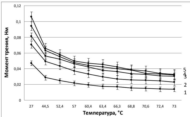
Рис. 5. Зависимость момента трения от температуры в рабочем зазоре, образованном сменной втулкой (сталь 3, Ra=1,220 мкм) и сменным полюсом (сталь 3; Ra=3,301 мкм) и заполненным магнитной жидкостью типа МКУ 100-40, с разными частотами вращения втулки: 1 – 556 об/мин; 2 – 1146 об/мин; 3 – 1793 об/мин; 4 – 2331 об/мин; 5 – 2897 об/мин
