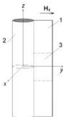
Рис.1. Схема ячейки. 1 – канал, 2- Ферром. стержень, 3 – область регистрации
