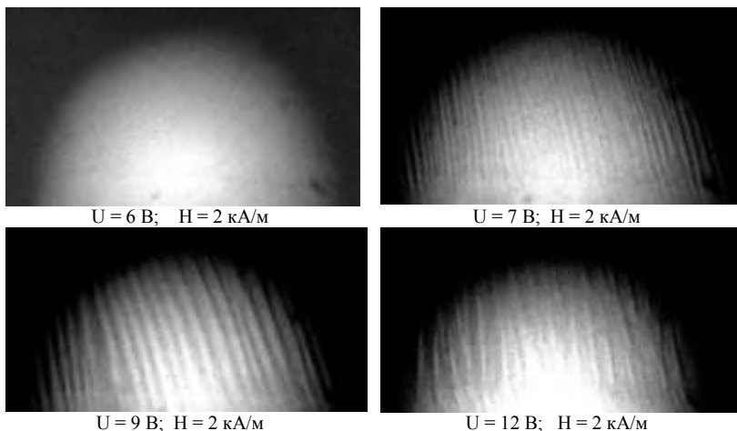
Рис.4. Пороговый характер формирования электрокапиллярной неустойчивости
