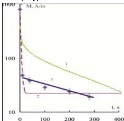
Рис. 3. Релаксация остаточной намагниченности образца №1: 1 – степенная функция; 2 – экспоненциальная; 3 – экспоненциальная без учета первой точки
