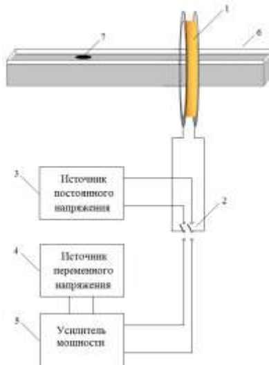
Рис. 1. Схема экспериментальной установки по изучению особенностей движения капли магнитной жидкости в неоднородном магнитном поле
