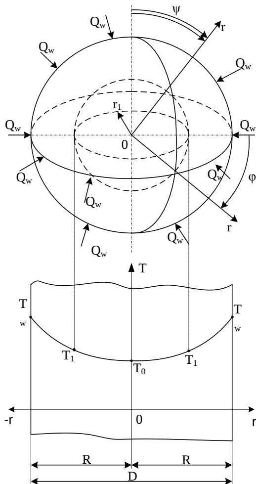
Рис. 1.3. Изотермические поверхности в шаре:
