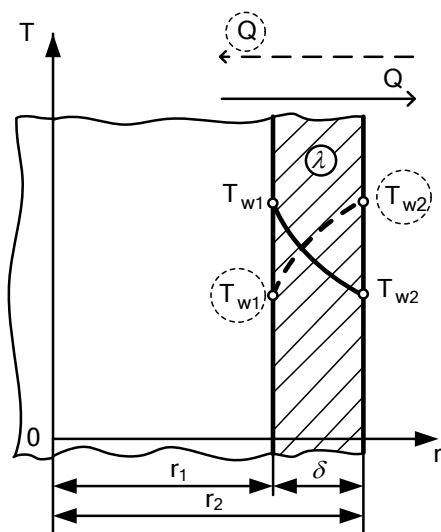
Рис. 2.2. Стационарное температурное поле в цилиндрической стенке
