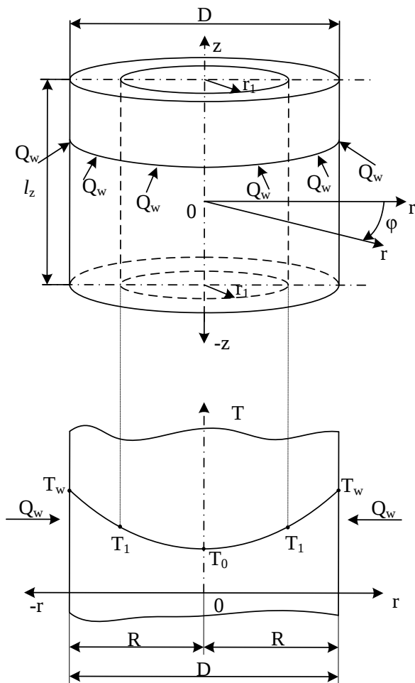
Рис. 1.2. Изотермические поверхности в бесконечном цилиндре:
