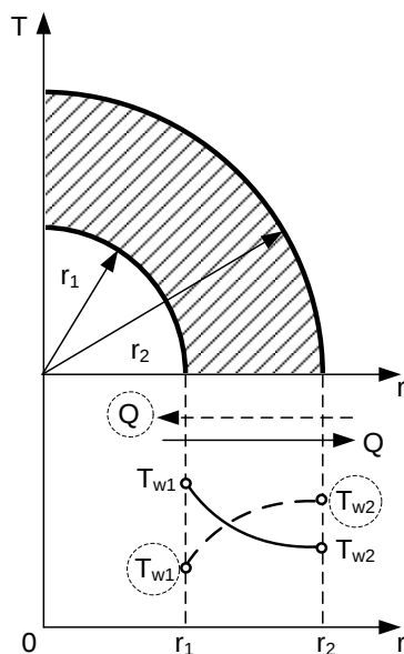
Рис. 2.3. Стационарное температурное поле в шаровой стенке
