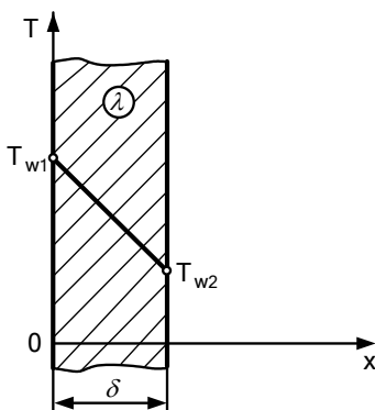
Рис. 2.1. Стационарное температурное поле в плоской стенке
