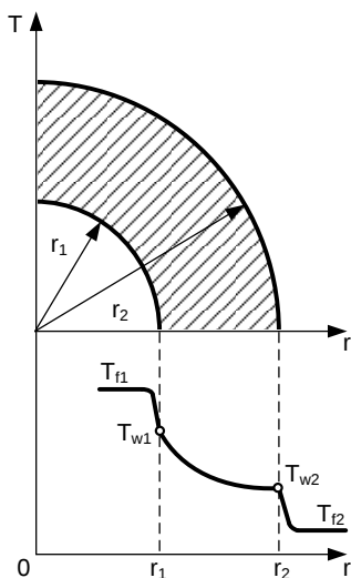
Рис. 2.6. Теплопередача через шаровую стенку
