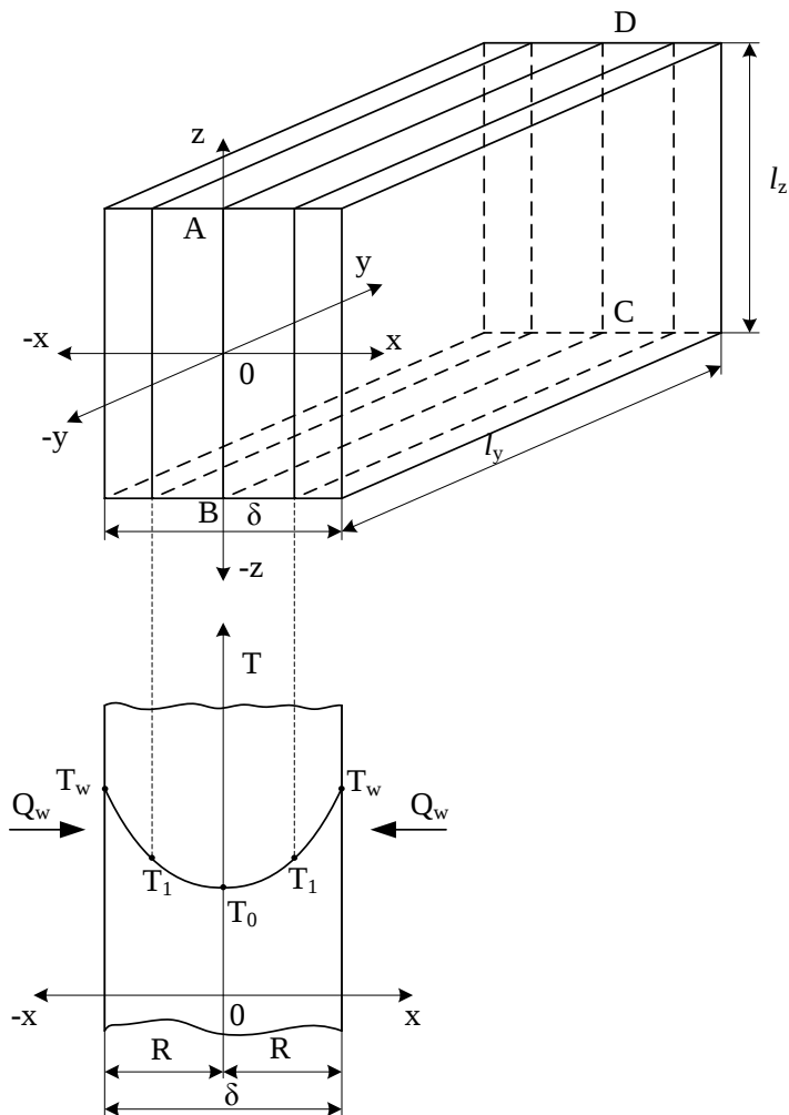
Рис. 1.1. Изотермические поверхности в бесконечной пластине:
