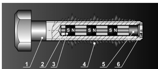
Рис. 2. Конструкция трибологически безопасного резьбового соединения «закрытого» типа: 1 – тело винта M20x2; 2 – кольцо проставное из магнитного материала; 3 – постоянный магнит; 4 – магнитная жидкость на основе полиэтилсилоксановой основе (ПЭС-5); 5 – проставка-цилиндр из магнитного материала; 6 – заглушка
