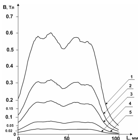
Рис. 6. Зависимость напряженности постоянного магнитного поля на рабочей поверхности винта от материала постоянного магнита, установленного в его теле: 1 – неодим-железо-бор N34A – 2706 кА/м; 2 – самарий-кобальт S24H – 1440 кА/м; 3 – неодим-железо-бор N34A – 2520 кА/м; 4 – альнико A5.05B – 147 кА/м; 5 – феррит F3.2c – 380 кА/м
